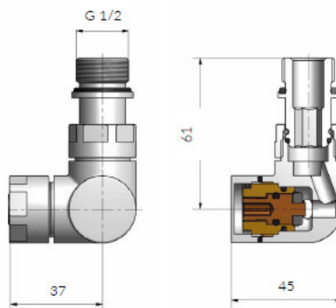
Zawór osiowy odcinający
