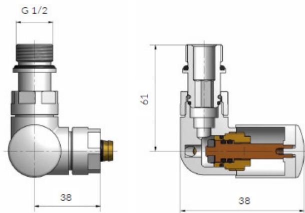
Zawór osiowy regulacyjny
