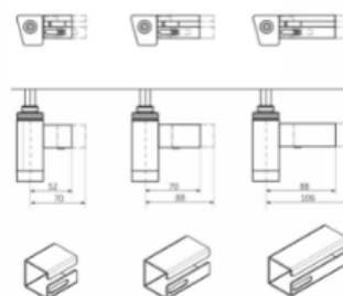
M - kabel prosty bez wtyczki z maskownicą (standardowa długość maskownicy: 52-70 mm)
