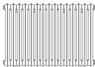
860 x 1262 15 sekcji
