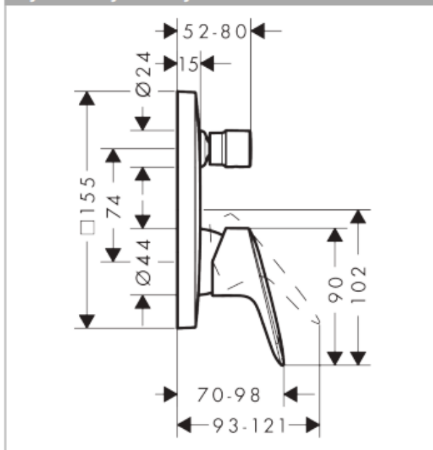
Rysunek wymiarowy
