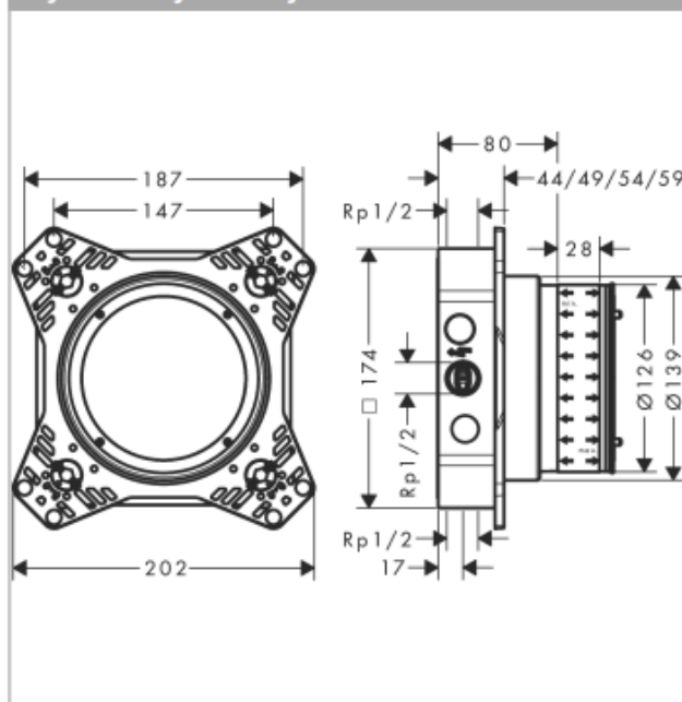
Rysunek wymiarowy
