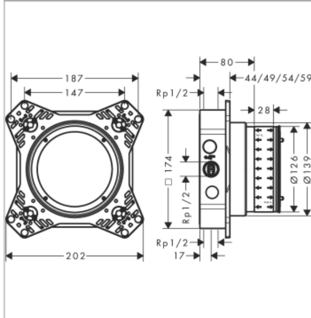
Rysunek wymiarowy
