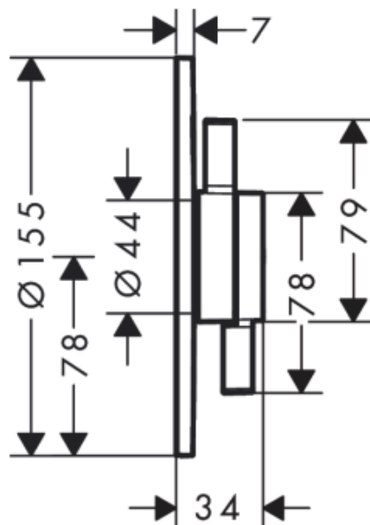
Rysunek wymiarowy
