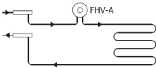
System ogrzewania podłogowego, pętla z zaworem FHV-A na zasilaniu
