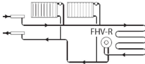
System ogrzewania podłogowego, mieszkaniowego z zaworem FHV-R na powrocie
