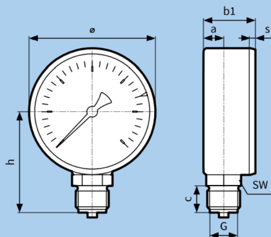
RF/HY/HZ 80 – przyłącze radialne
