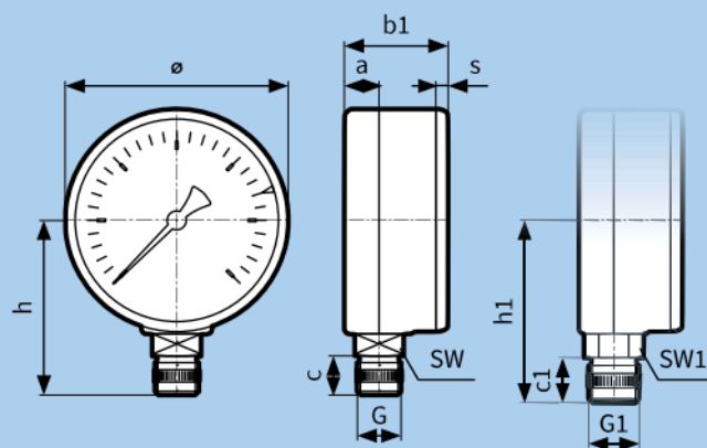
RF/HY/HZ 80 – przyłącze radialne
