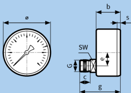
HZ 50 – przyłącze ekscentryczne
