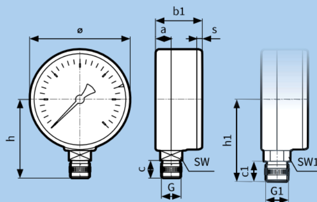
RF/HV/HZ 80 – przyłącze radialne
